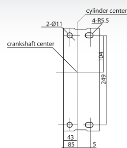
Ingombro basamento
