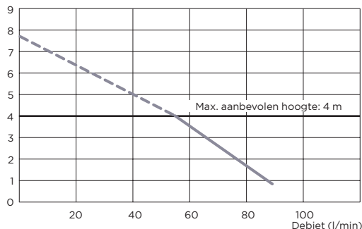
Opvoerhoogte (m)
