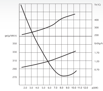
Diagramma consumo e potenza
