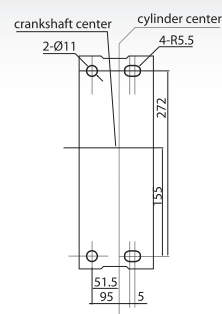
Ingombro basamento
